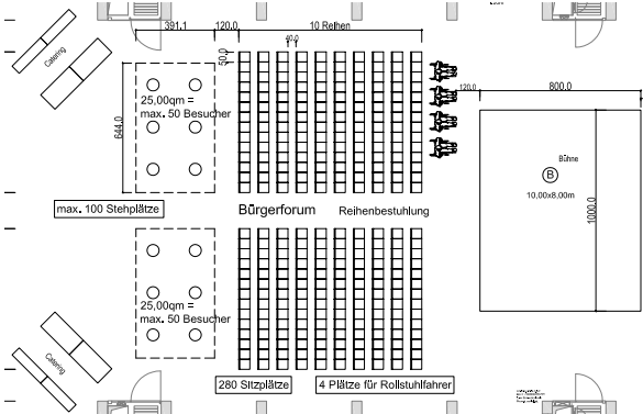
Reihenbestuhlung und Catering im Bürgerforum
