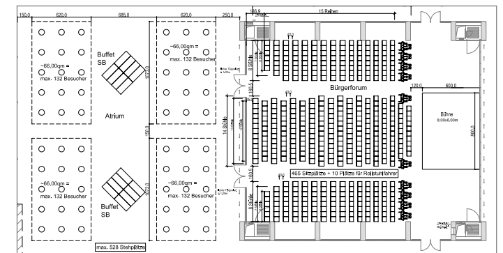
Reihenbestuhlung im Bürgerforum und im Atrium
