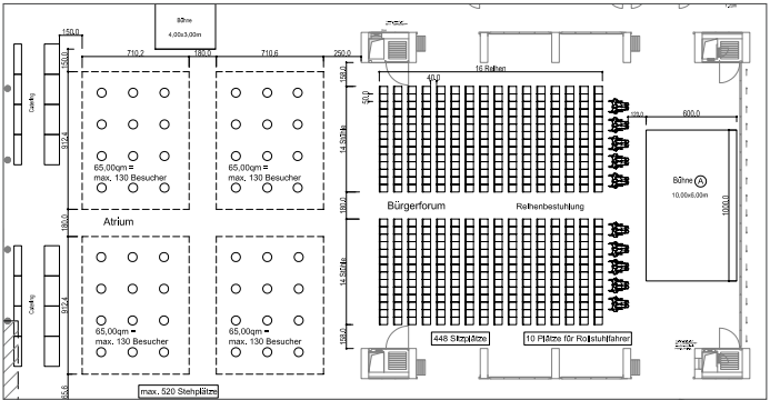
Reihenbestuhlung im Bürgerforum, „GET TOGETHER“ im Atrium
