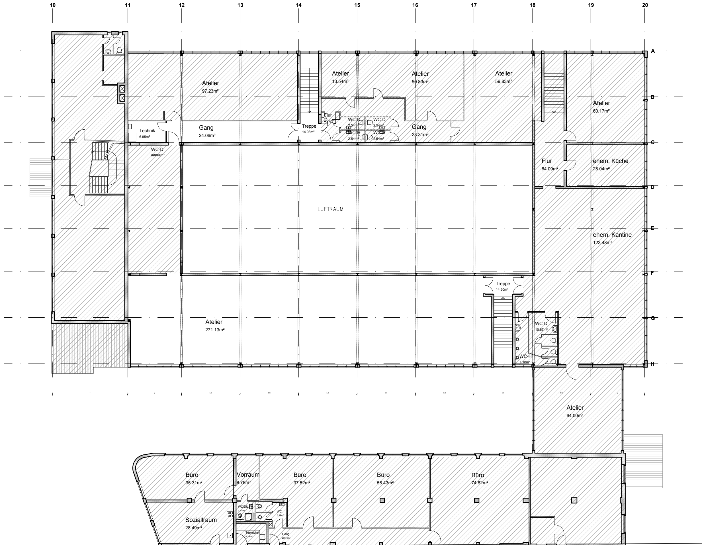
GRUNDRISS OBERGESCHOSS HAUS HALLE HEDDERNHEIMER LANDSTRASSE 155 60439 FRANKFURT/M. DIN A3 PLANUNGSSTAND 17.11.22 M: 1:200
