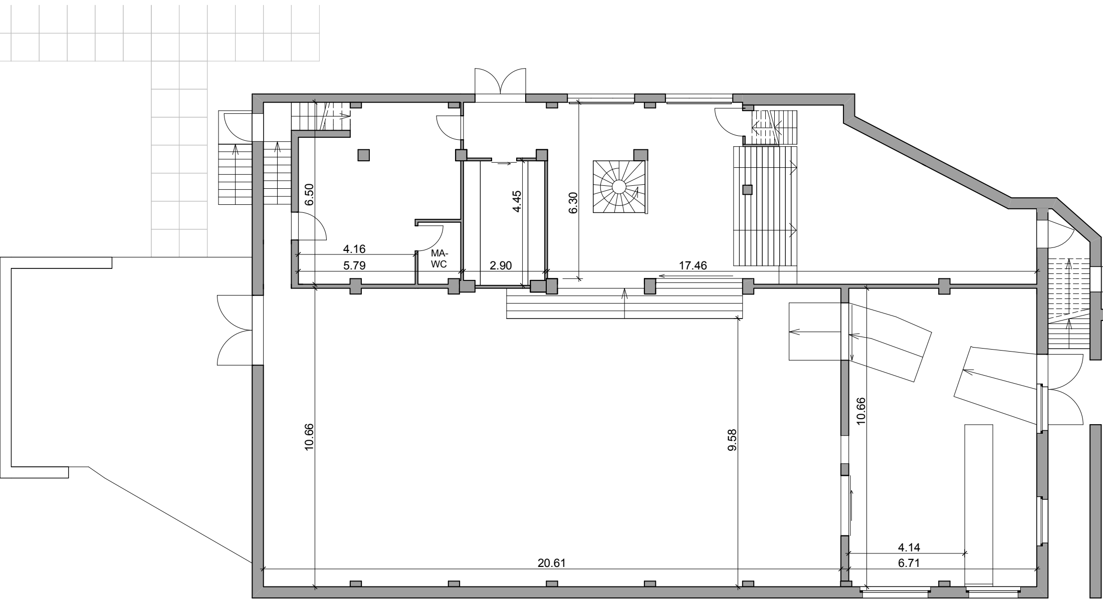
Stufenbau Eventlocation - Eventplan - Grundriss 5. Obergeschoss
