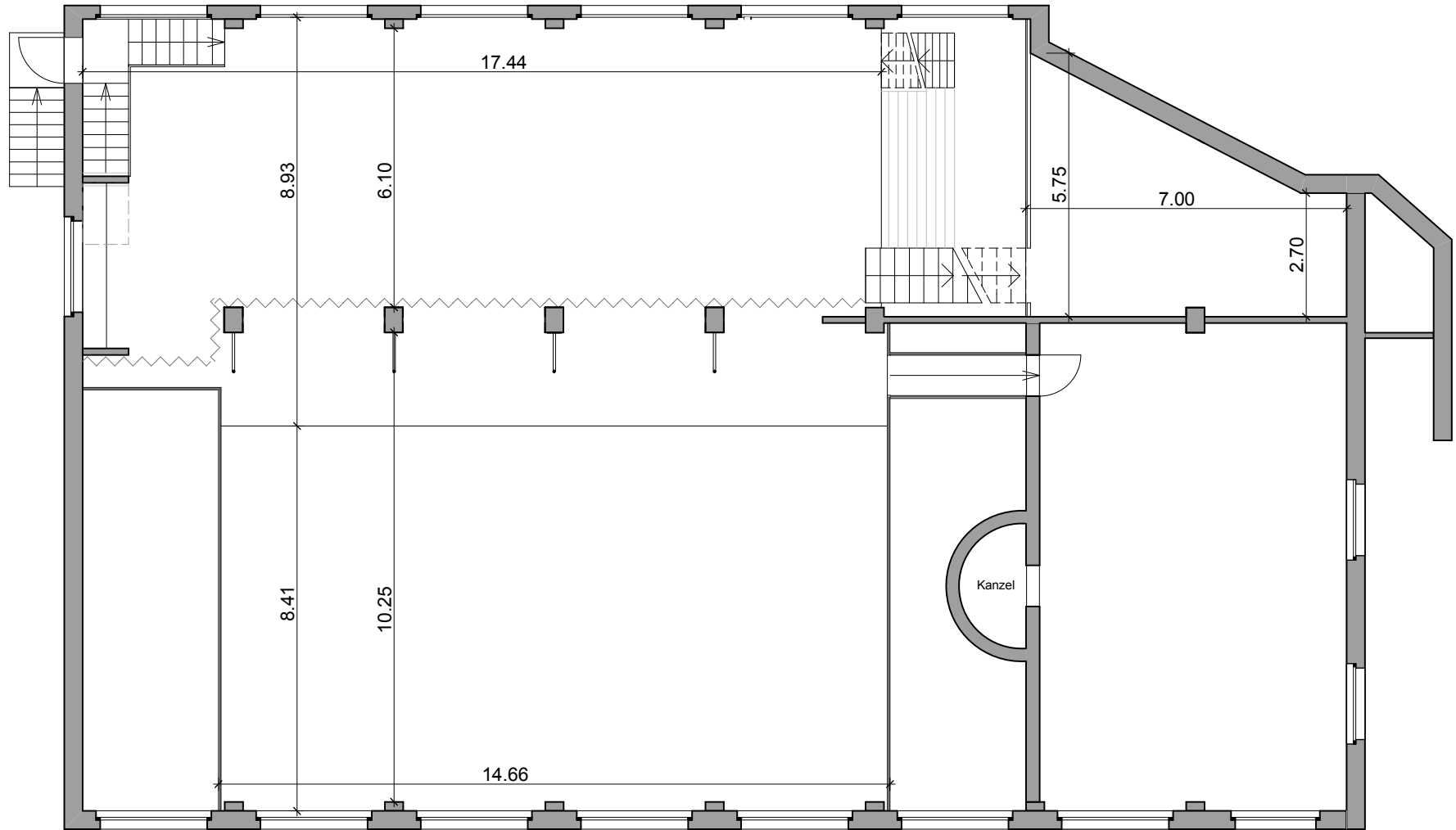
Stufenbau Eventlocation - Eventplan - Grundriss 6. Obergeschoss
